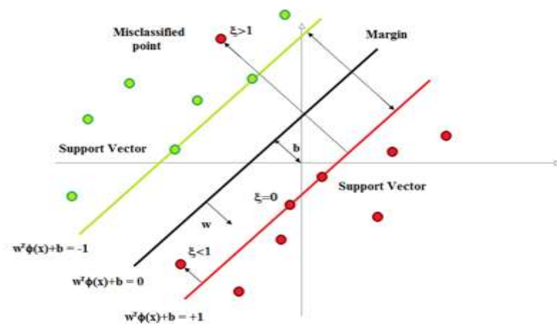
شکل ۲: نمایی از ماشین بردار پشتیبان
