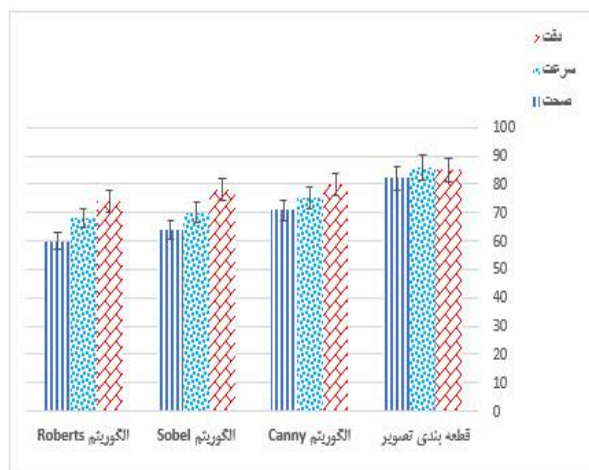
نمودار ۱: مقایسه دقت و سرعت و صحت روش پیشنهادی با سایر روش ها
