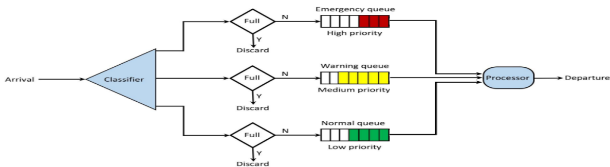
شکل ۲: طبقه‌بندی درخواست‌ها در صف‌های اولویت لایه مه
