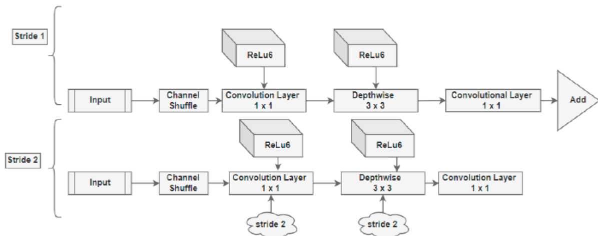
شکل ۴: تصویر شماتیک معماری MobileNet-v2 مورد استفاده در مطالعه [۲۶]
