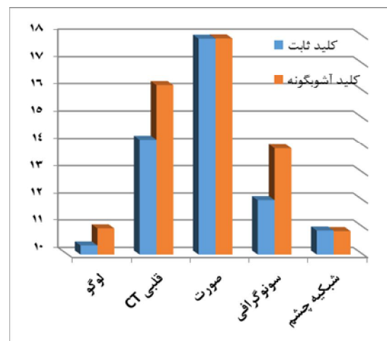
نمودار ۴: نسبت پیک سیگنال به نویز میان دو تصویر رمز نشده و رمزگشایی شده توسط کلید نادرست توسط الگوریتم های رمزنگاری راین دال با کلید ثابت و متغیر آشوب گونه
