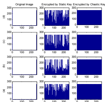
شکل ۹: هیستوگرام‌های تصاویرهای لوگو قبل و بعد از رمزنگاری با کلیدهای متفاوت (ستون‌ها به ترتیب از سمت چپ، تصویر رمز نشده، رمز شده با کلید ثابت و رمز شده با کلید آشوب‌گونه)
