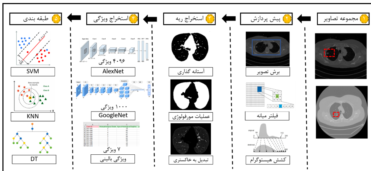
شکل ۱: شمای کلی روش پیشنهادی. (۱) جمع‌آوری داده (۲) پیش‌پردازش (۳) ناحیه بندی تصویر جهت استخراج ناحیه ریه (۴) استخراج ویژگی (۵) طبقه بندی توسط روش‌های SVM، KNN و DT
