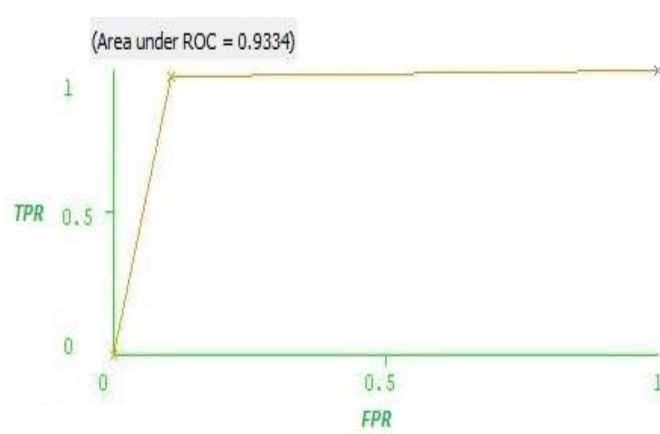
SVM
